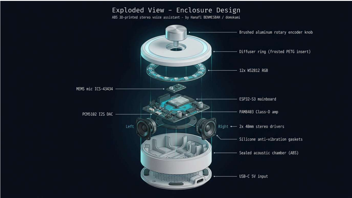
Fig. 5 - Exploded view de l'enclosure, composants et finition.
